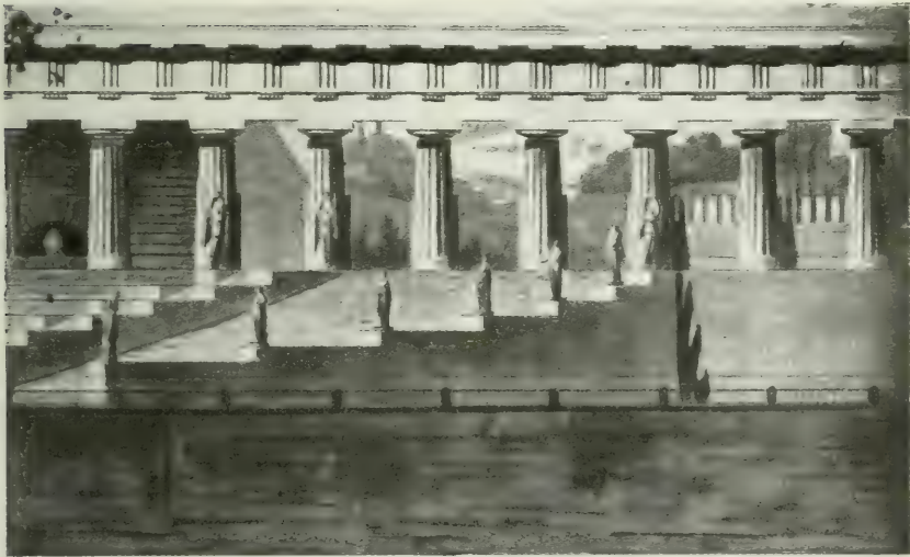
COLONNADE AU BORD DE LA MOSKVA WITBERG. — PROJET DE L'ÉGLISE DU SAUVEUR A MOSCOU.
